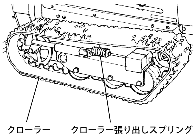
クローラー張り出しスプリング部詳細
